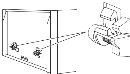
фиксатор (блокирование)
